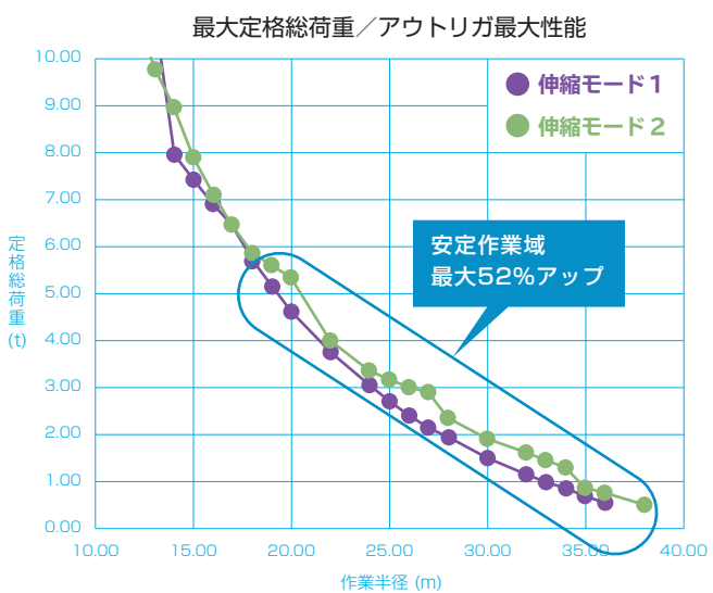
伸縮モード1 [2段目・3段目ブーム先伸長方式] 伸縮モード2 [4段目・5段目・トップブーム先伸長方式]
