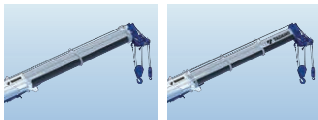
伸縮モード1 [2段目・3段目ブーム先伸長方式] 伸縮モード2 [4段目・5段目・トップブーム先伸長方式]
